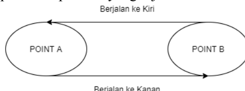
Gambar. 4. FSM musuh
