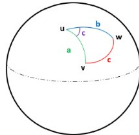
Gambar. 1. Pola Haversine
