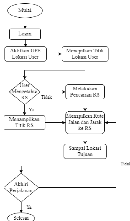
Gambar. 3. Flow Chart Aplikasi
