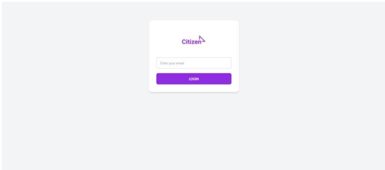
Gambar 6. Halaman Login
