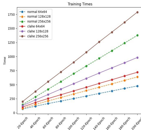
Gambar 211. Grafik Waktu Training
