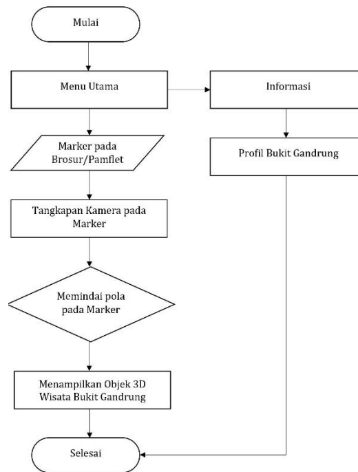
Gambar 2. Flowchart Aplikasi Gandrung Plus
