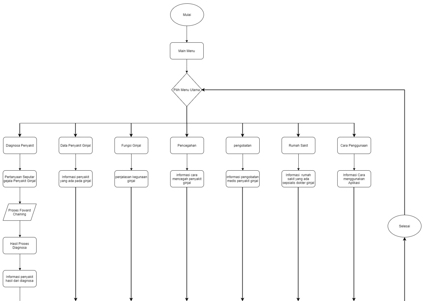
Gambar. 3. Flowchart Aplikasi
